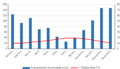
Fig. 7. Climograma para la ciudad de Muros según el estándar del índice Xerotérmico de Gausson, dónde la escala de las precipitaciones debe ser el doble que la de la temperatura.
