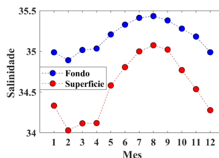
Fig. 16. Variación intra-anual de la salinidad en la estación M3 "A Creba" (parte interna del estuario) para el período 2006-2018. Línea azul promedio a los tres últimos valores de la columna de agua y línea roja promedio a los tres primeros.
