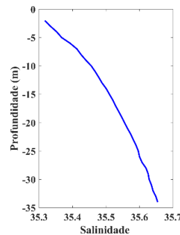
Fig. 23. Perfil vertical de salinidad media para el periodo 2006- 2018 en la estación M8 "As Bazoñas" (boca sur del estuario).
