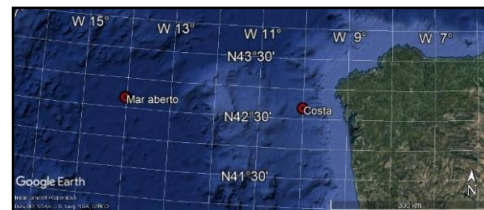
Fig. 4. Localización de los puntos de extracción de los datos de SST.
