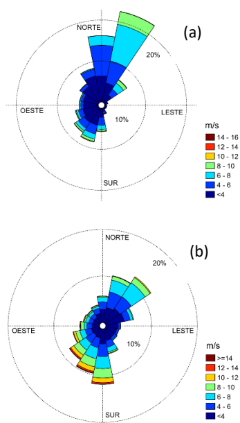
Fig. 9. Rosa de los vientos para un punto situado enfrente de la boca de la Ría de Muros y Noia ( 42^{\circ} 42'N , 9^{\circ}12' W ) para el periodo 1982- 2017 mostrando, la velocidad en m/s, la frecuencia en porcentaje y la dirección del viento para el periodo (a) de abril a septiembre y (b) octubre a marzo.
