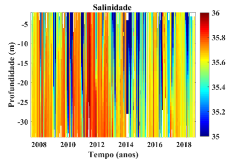
Fig. 22. Variación interanual de la salinidad de la columna de agua en la estación M8 "As Bazoñas" (boca sur del estuario).
