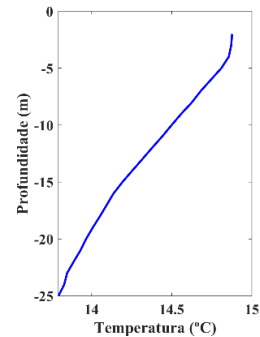
Fig. 31. Perfil vertical de temperatura media para el periodo 2006-2018 en la estación M4 "Centro ría".
