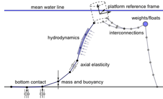
Fig. 2. Modelo de MoorDyn
