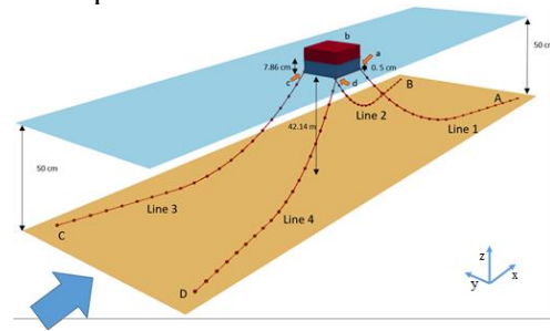
Fig. 4. Configuración del experimento realizado por la Universidad de Gante.
