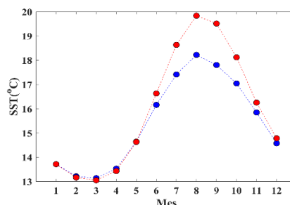
Fig. 11. SST mensual media para un punto próximo a la costa ( 42^{\circ} 42'N , 10^{\circ} W , línea azul) y un punto en el océano ( 42^{\circ} 42'N , 14^{\circ} W , línea roja).
