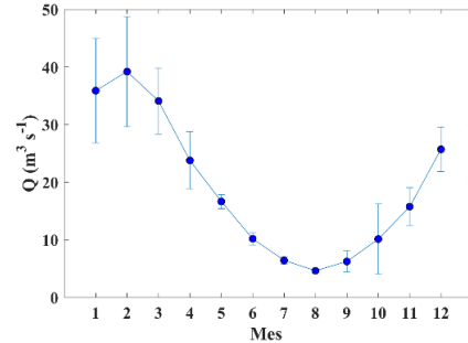
Fig. 5. Variación intra-anual del caudal del río Tambre para el período 2010- 2018.
