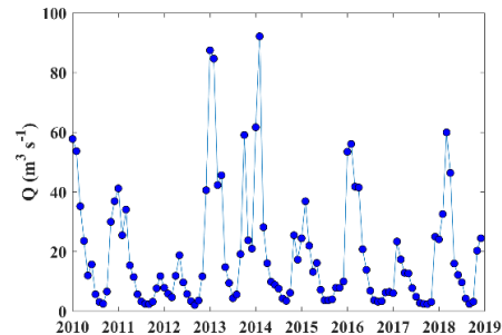
Fig. 6. Variación inter-anual del caudal mensual del río Tambre para el período 2010- 2018.
