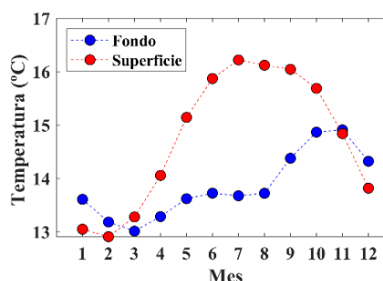
Fig. 34. Variación intra-anual de la temperatura en la estación M4 "Centro ría" para el periodo 2006- 2018. Línea azul promedio a los tres últimos valores de la columna de agua y línea roja promedio a los tres primeros.
