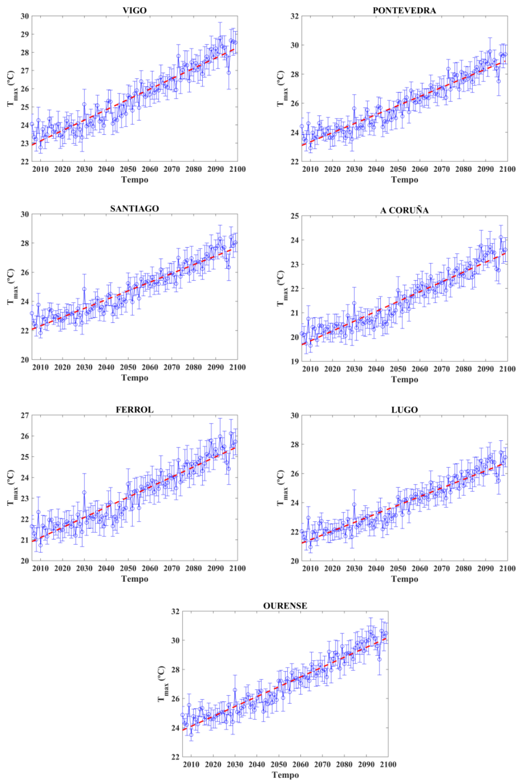
Fig. 4. Gráficas da variación da temperatura máxima elaborados a partir dun promedio de RCMs de CORDEX (°C) para o período 2006-2099 nas 7 cidades principais galegas.
