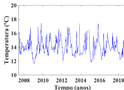
Fig. 37. Variación interanual de la temperatura media de la columna de agua en la estación M8 "As Basoñas" (boca sur del estuario).
