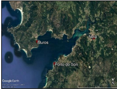
Fig. 3. Localización de las ciudades para las que se extrajeron los datos de los climogramas.
