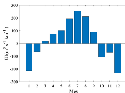
Fig. 10. Índice de afloramiento calculado para un punto en frente de la Ría de Muros y Noia ( 42^{\circ} 42'N , 9^{\circ}12' W ) para el periodo 1982- 2017.
